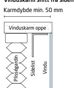
Vinduskarm snitt fra siden
