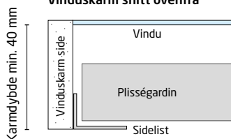
Vinduskarm snitt ovenfra
