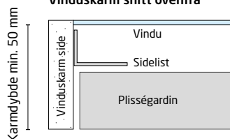
Vinduskarm snitt ovenfra
