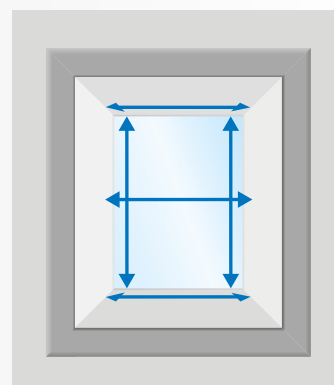
Figur 2. Montering i vindusramme/nisje.
